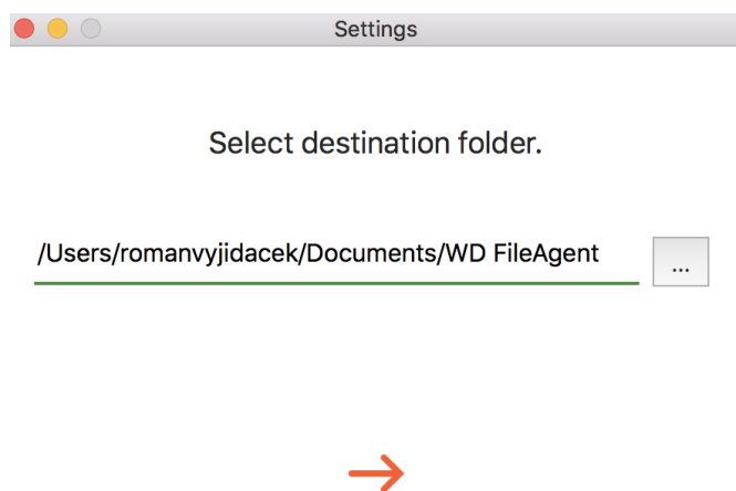
Obrázek 9: Výběr adresáře
