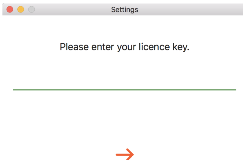
Obrázek 7: Zadání licence
