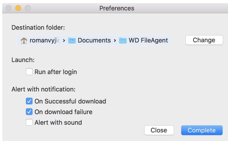
Obrázek 14: Předvolby
