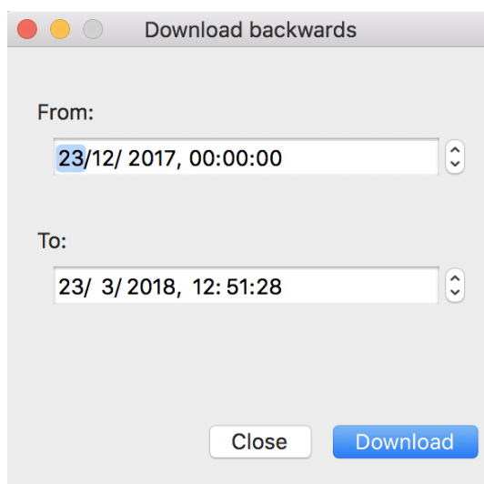
Obrázek 13: Zpětná synchronizace
