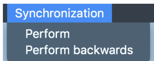
Obrázek 12: Menu-Synchronizace
