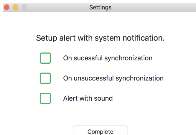
Obrázek 10: Zapnutí notifikací
